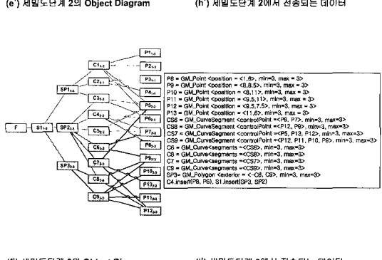
(B) 요소선택 세밀도 예제
