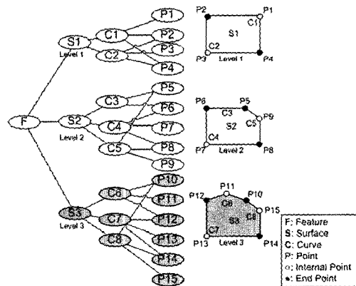
[그림 3] Separated LOD data model
